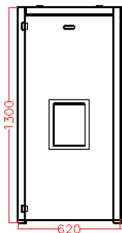
Fronte
